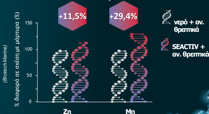
Μέτρηση της περιεκτικότητας Zn και Mn στο άνω τρίτο των φύλλων, 24 ώρες μετά τον ψεκασμό στο κάτω τρίτο
